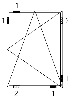
Наклонно-поворотная (поворотно-откидная) створка
